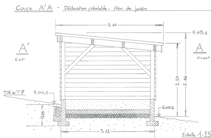
exemple pour un abri de jardin (voir emplacement coupe A'A sur plan de masse)
